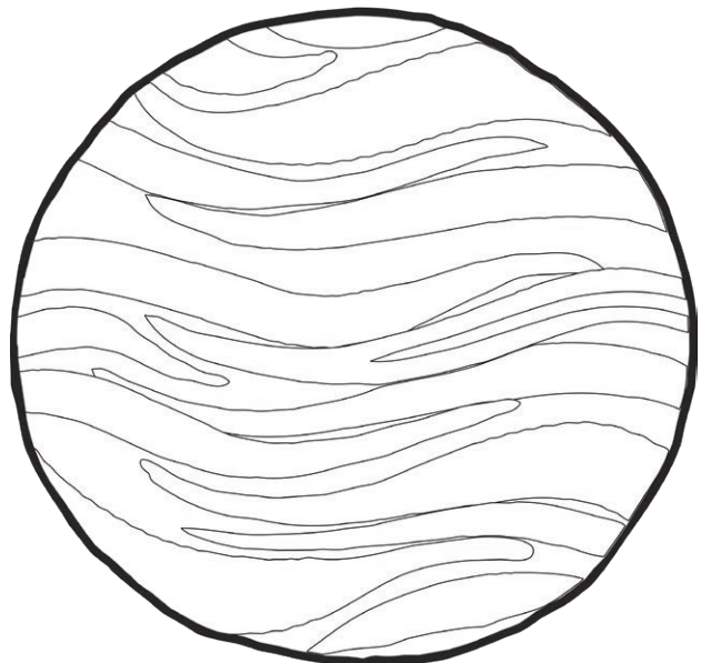
Jupiter
