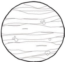
Venus
