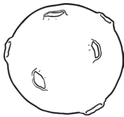
Mars
