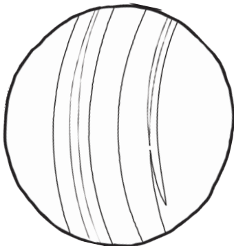
Uranus
